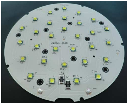
図 3 LED 基盤
