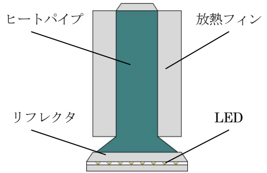
図 4 筐体断面図
