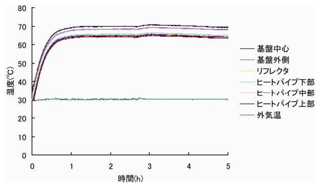
図 7b 放熱性能試験結果(0-5 h)
