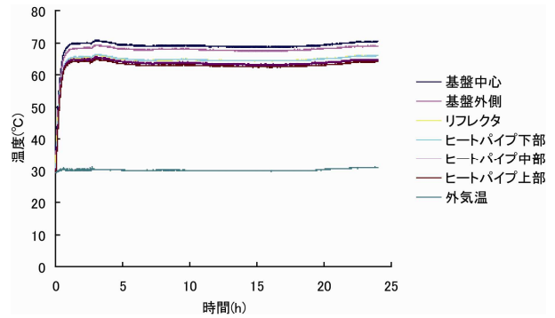
図 7a 放熱性能試験結果(0-24 h)
